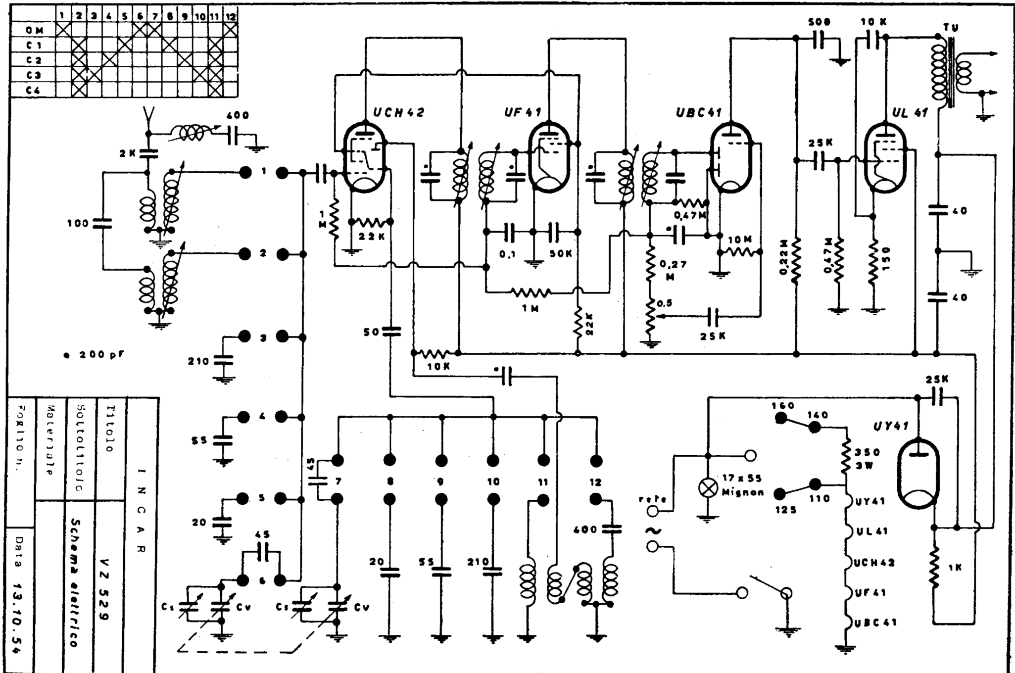
INCAR - Mod. VZ 529 - Ricevitore a onde medie con quattro bande allargate ad onde corte. Potenza d'uscita 3 watt. Consumo 50 watt.
